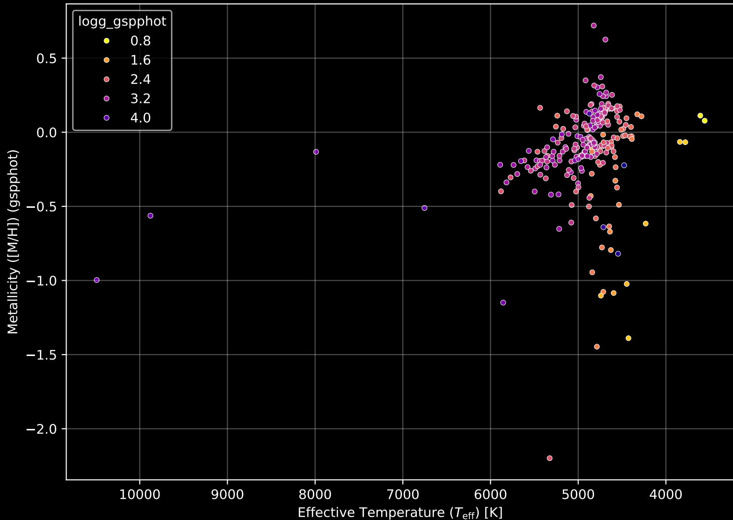
APOGEE DR17 Field: [355+08] Stellar Population Parameters (n= 242)
